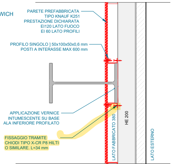
SEZIONE ORIZZONTALE - POST OPERAM
