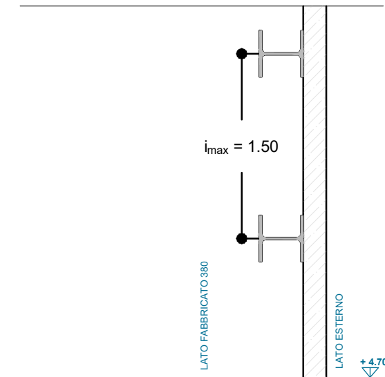
SEZIONE VERTICALE - ANTE OPERAM
