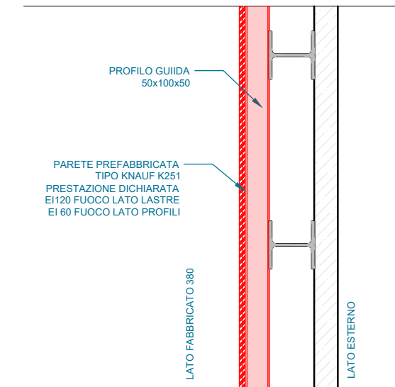
SEZIONE VERTICALE - POST OPERAM
