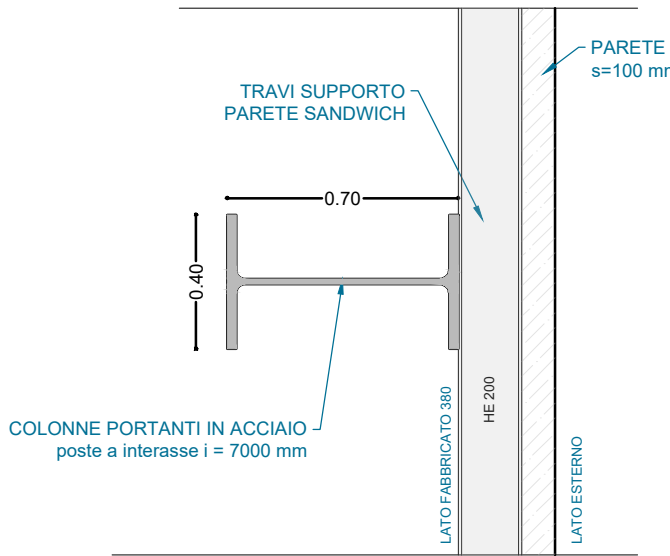
SEZIONE ORIZZONTALE - ANTE OPERAM
