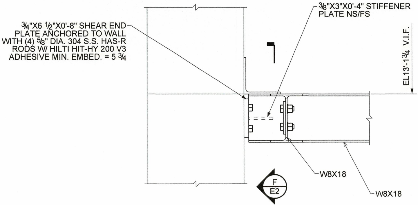
3 E2 DETAIL
