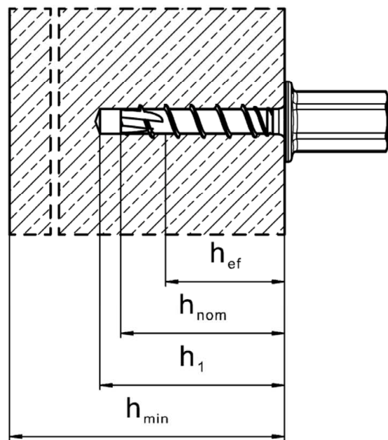
HUS3-I (Größe 6, Ausführung Sechskantkopf mit Innengewinde M8/M10)
