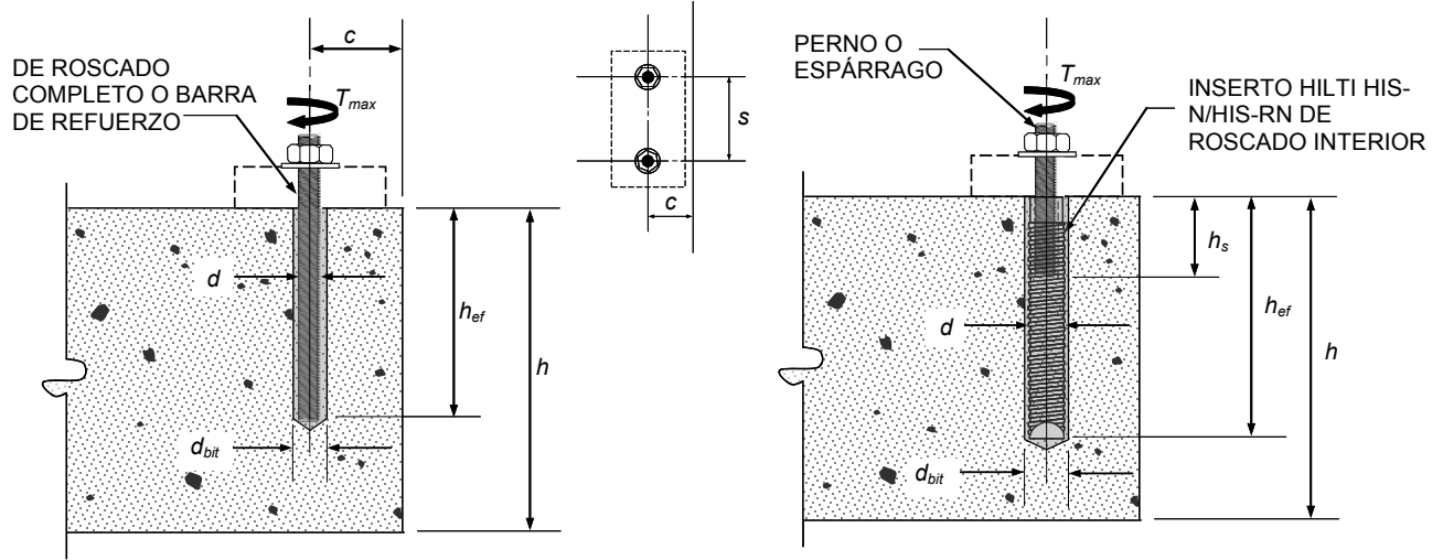
VARILLA ROSCADA/BARRA DE REFUERZO
