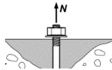
Resistencia al Arrancamiento del Concreto
