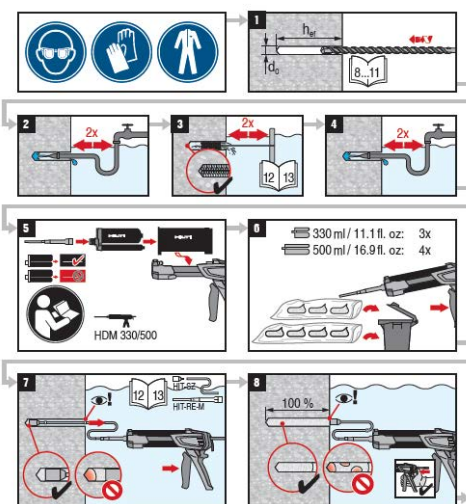
FIGURE 9A—INSTRUCCIONES DE INSTALACIÓN IMPRESAS Y PROPORCIONADAS POR EL FABRICANTE (MPII) (Continuación)
