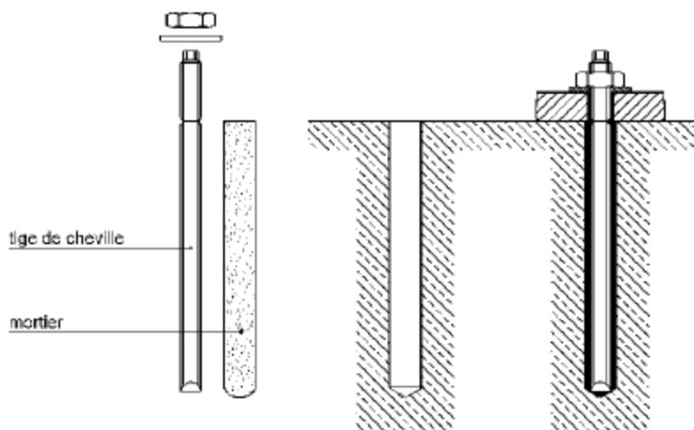
d) Exemple de chevilles à scellement (5 e partie)
