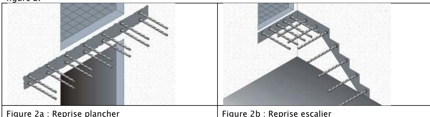
Figure 2 : Exemples de conception béton armé
