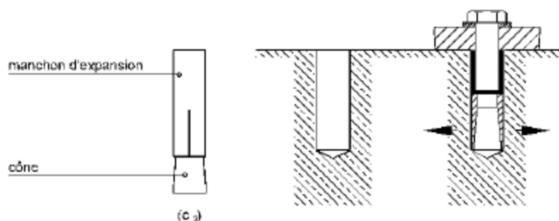
c) Exemple de chevilles à expansion par déformation contrôlée (4 e partie)
